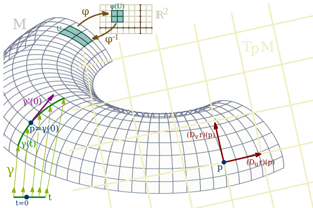
Abbildung 1: Torus
