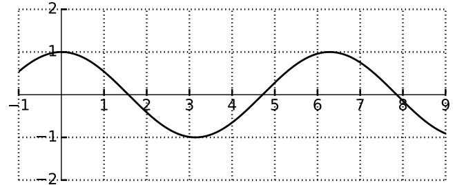
Abbildung 2.2: y = \cos(x)
