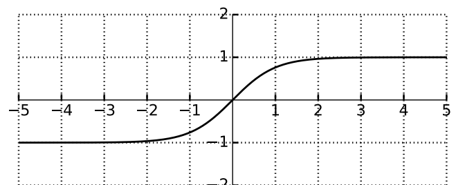
Abbildung 2.4: y = \tanh(x)
